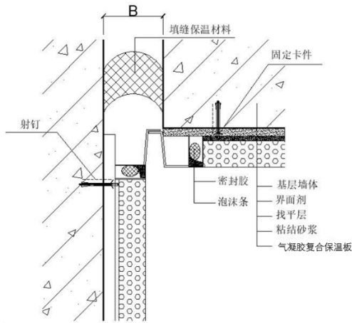
图 5.3.13-2 转角缝
