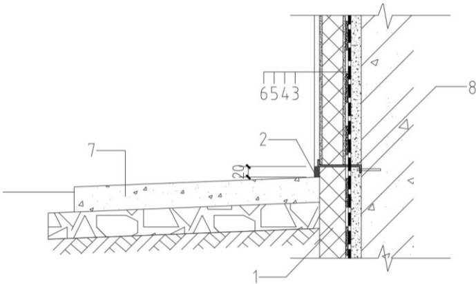
图 5.3.11 勒脚
