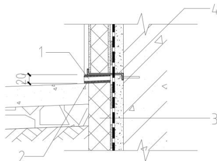
图 5.3.6 排水管
