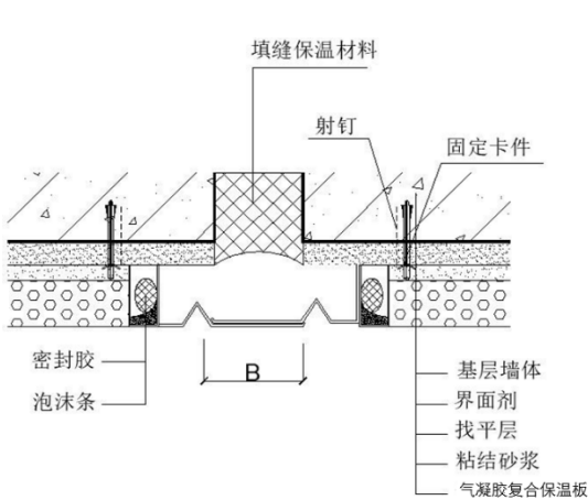
图 5.3.13-1 平缝
