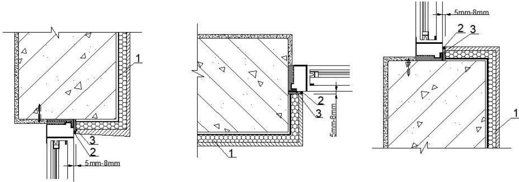
图 5.3.9-1 窗上口
