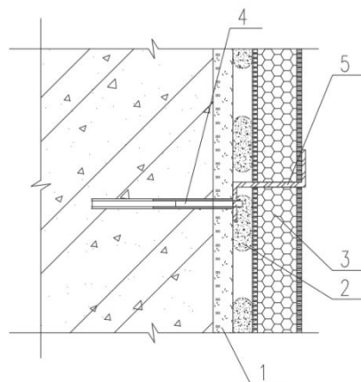
图 5.3.7 板缝
