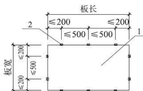
图 5.3.4-1 固定卡件设置示意图
