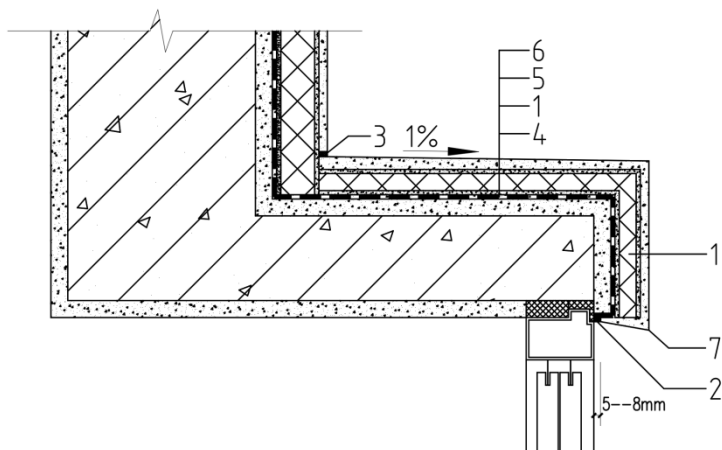
图 5.3.12 凸窗顶
